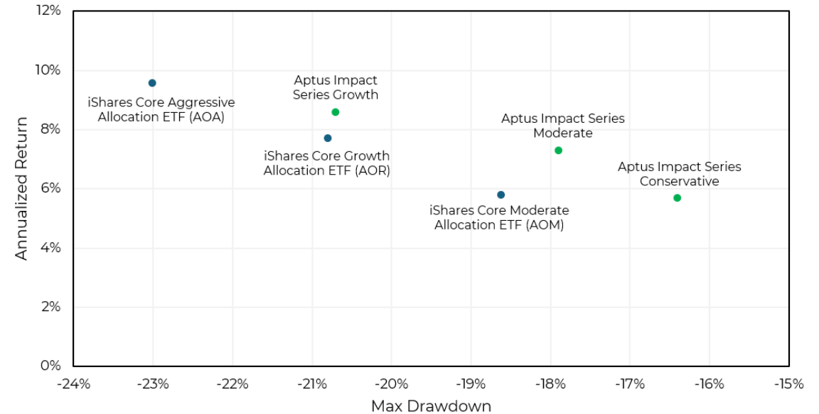
Return vs Max Drawdown 01.01.2017 - 06.30.25
